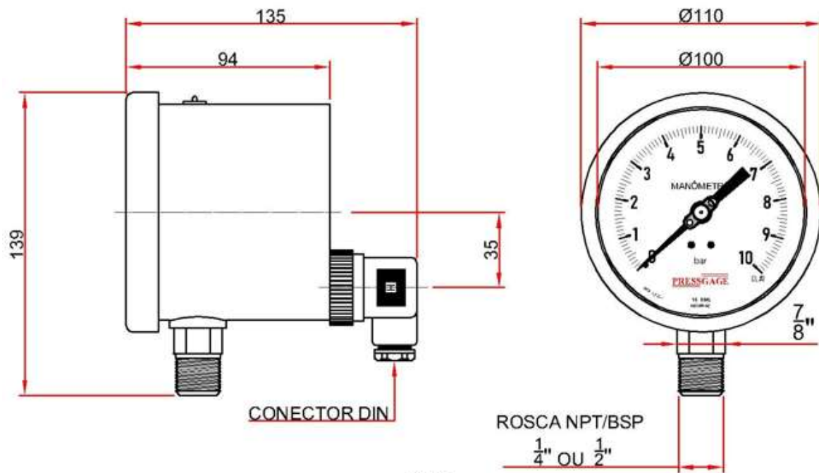
Figura 1: Manômetro analógico Ø100mm com transmissão de sinal
